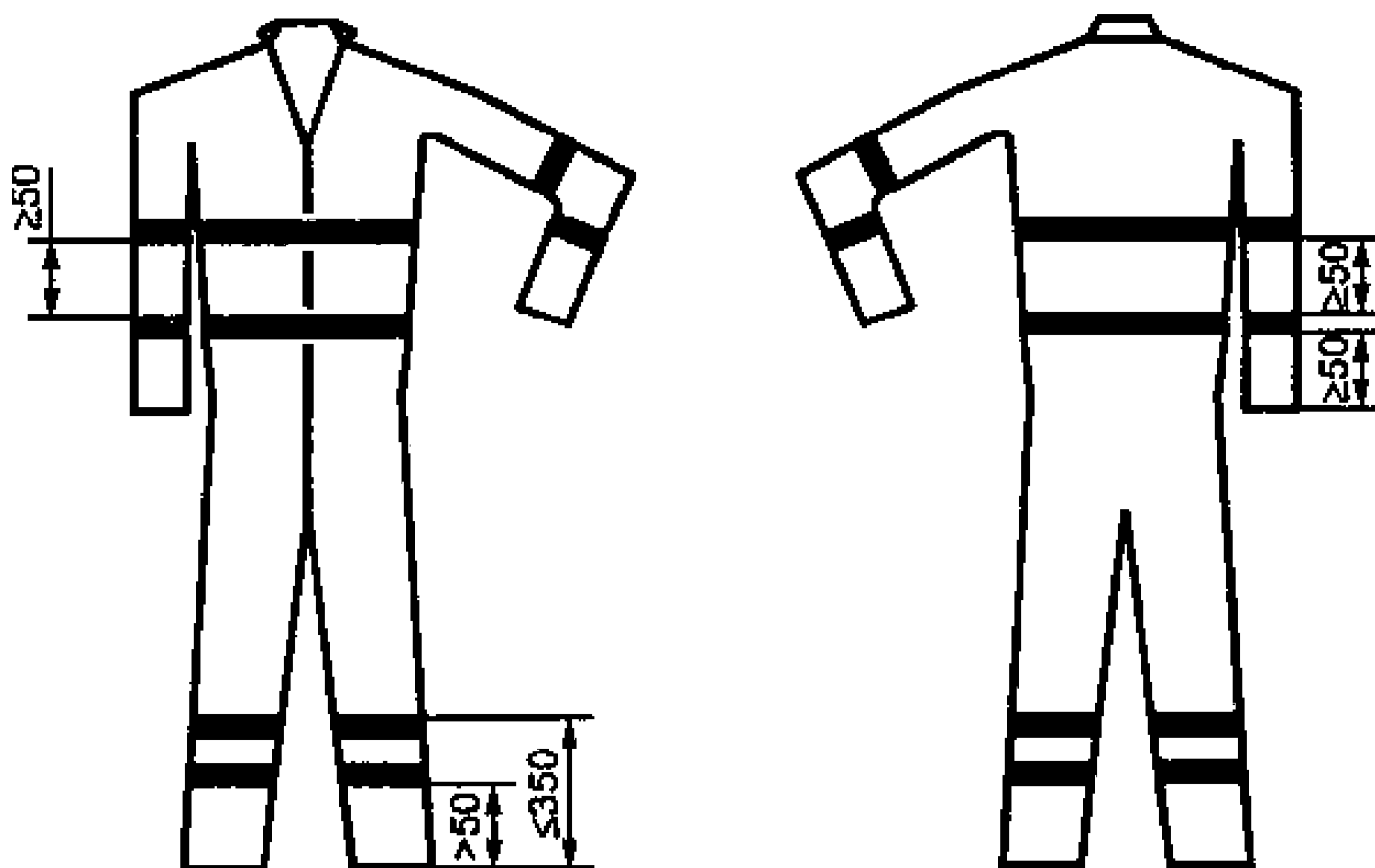
Рисунок Б.1 – Закрытый комбинезон
