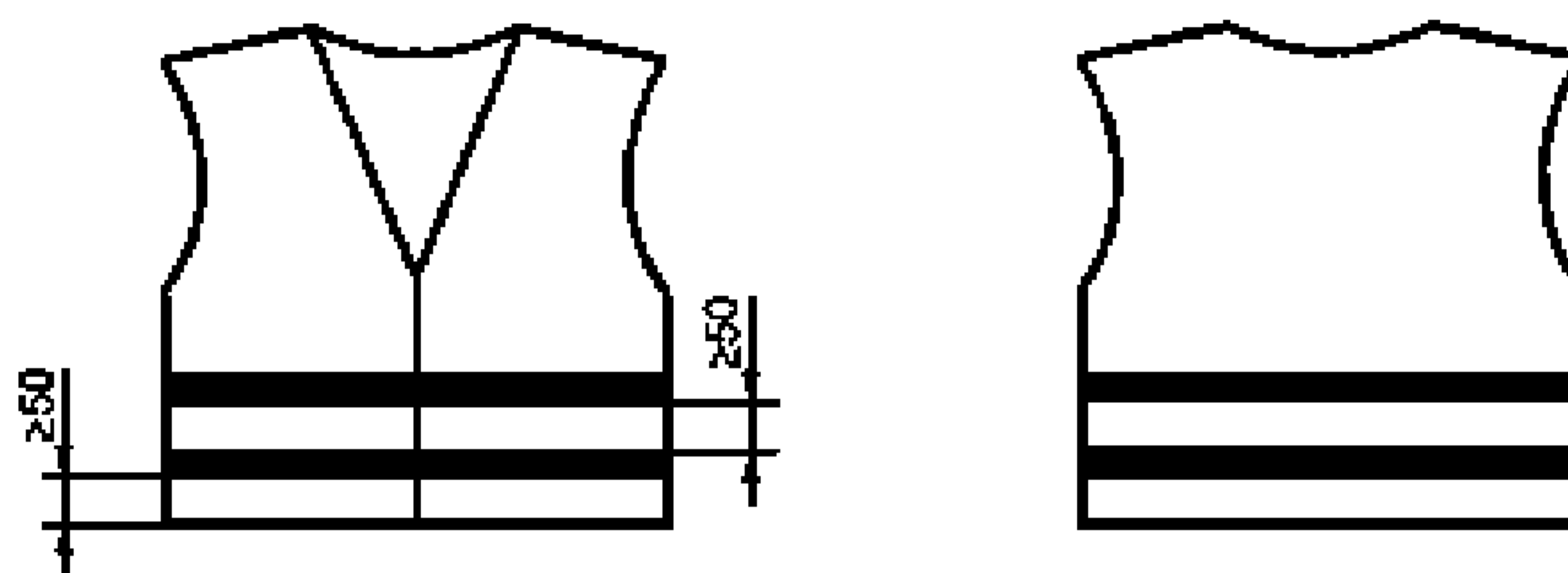
Рисунок Б.3 – Жилет-1
