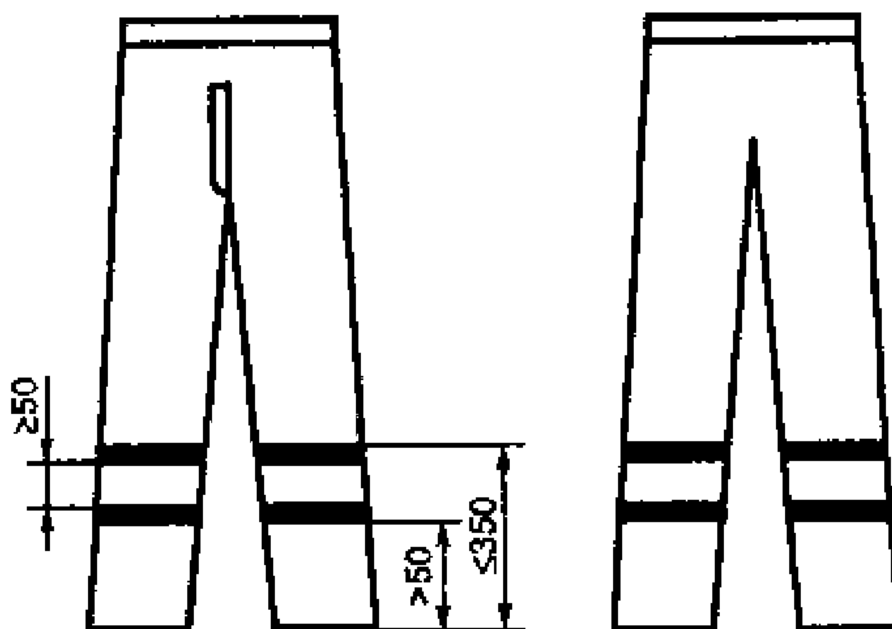
Рисунок Б.9 – Брюки
