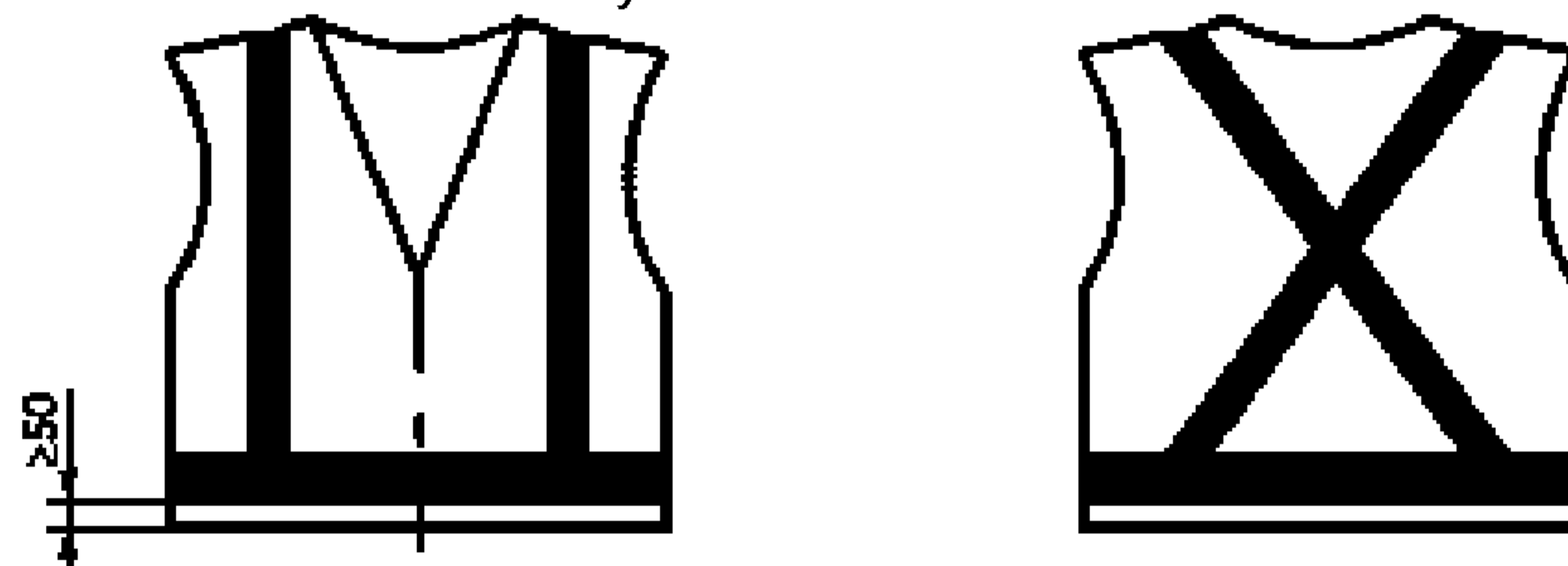
Рисунок Б.4 – Жилет-2
